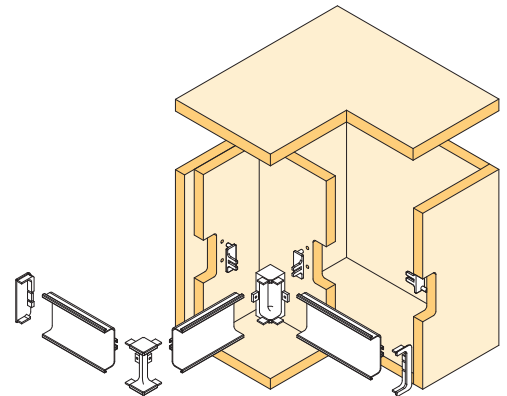
Profil uchwytowy poziomy „C”
