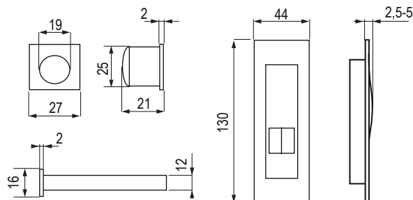
frezowany otwór głębokość: 11 mm
