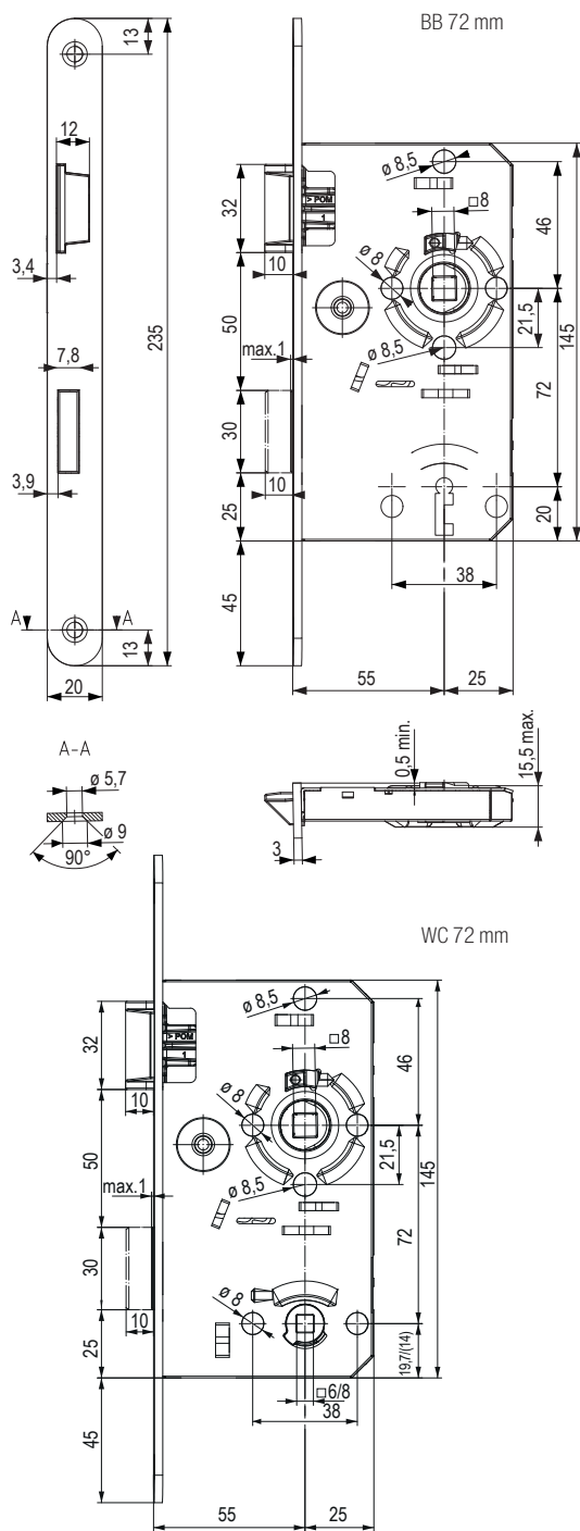
plastikowy zaczep BB/72 mm
