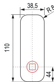
frezowany otwór głębokość: 11 mm
