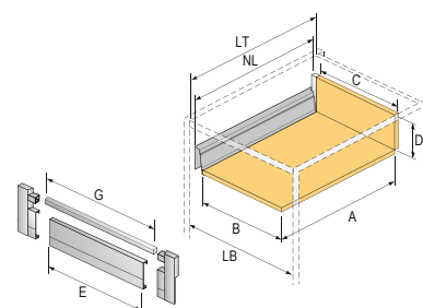
Wewnętrzna szuflada, wysokość 70 / 144 mm
