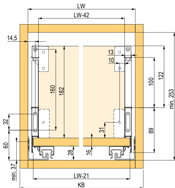
StrongMax podniesiona ścianka boczna 89 mm
