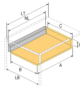
Przednia szuflada, wysokość 54 mm
