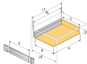
Wewnętrzna szuflada, wysokość 70 mm
