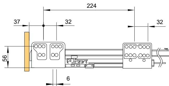
wiercenie otworów dla długości od 350 mm do 550 mm
