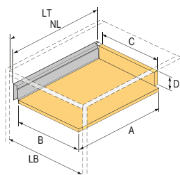
Wewnętrzna szuflada, wysokość 70 mm
