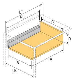
Wewnętrzna szuflada, wysokość 70 / 144 mm
