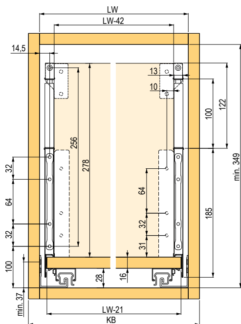
StrongMax podniesiona ścianka boczna 185 mm
