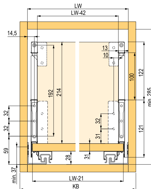
StrongMax podniesiona ścianka boczna 121 mm
