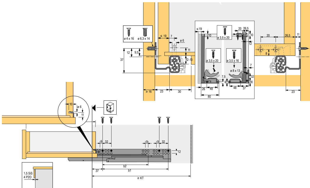
Prowadnica pełnego wysuwu Quadro V6
