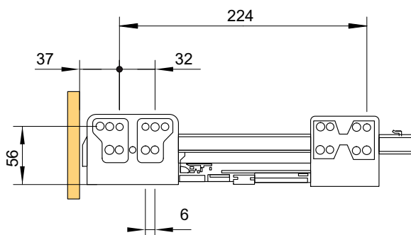
wiercenie otworów dla długości 270 mm i 300 mm
