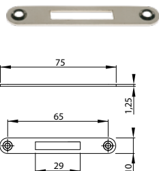
Płytkę zaczepową
