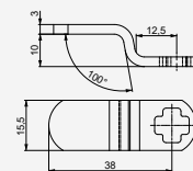
309277 język blokujący 400 wygięty
