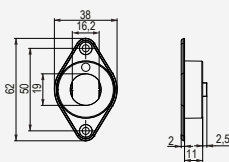
309274 adapter do montażu w drewnie
