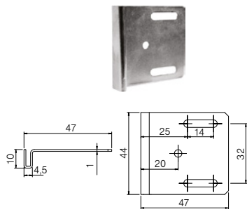
Kątownik 44 mm
