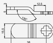
309276 język blokujący 390 zakrzywiony
