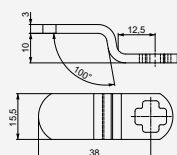
309277 język blokujący 400 zakrzywiony
