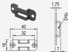
Prowadnica drążka
