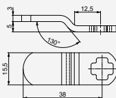
309276 język blokujący 390 wygięty
