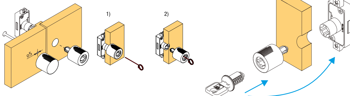
sposób wyciągania gałki z zamka
