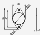
350805 podkładka plastikowa do montażu do cienkiego materiału, do połączenia z adapterem 309274
