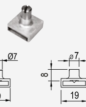
Zaczep drążka wraz z mocowaniem
