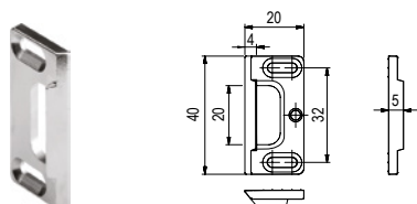
Kątownik zamka 584
