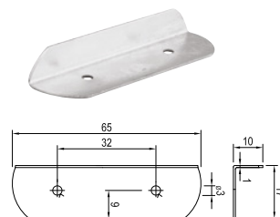
Kątownik 65 mm
