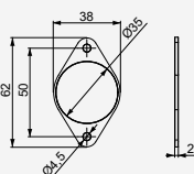
350805 wkładka plastikowa do montażu do cienkiego drewna, należy połączyć z adapterem 309274
