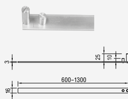
Drążek
