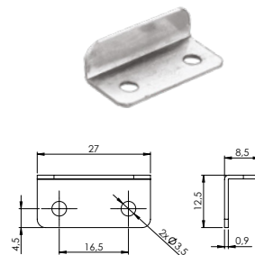
Kątownik 27 mm
