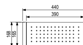
487892 | Wkład ociekowy ze stali nierdzewnej /z plastiku, przeznaczony do zlewozmywaków: 482139, 482140, 482141, 482144
