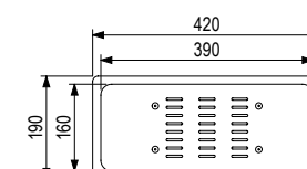
487891 | Wkład ociekowy ze stali nierdzewnej przeznaczony do zlewozmywaków: 482141, 482142, 482143, 482144
