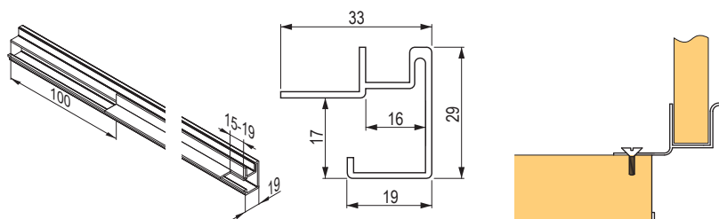
Rysunek skrócenia prowadnicy
