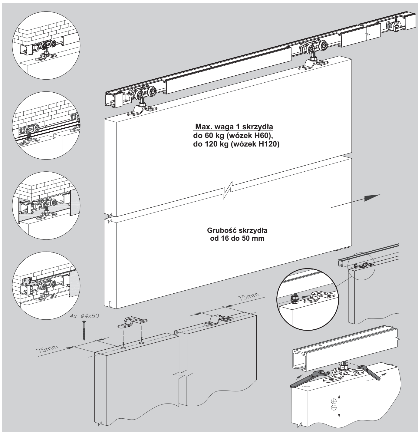
Prowadnica Herkules 2
